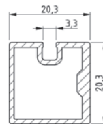
PROFIL ZA DRSNA VRATA SLIDING DOOR PROFILE
