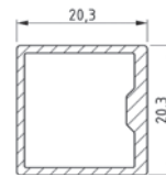
HORIZONTALNI PROFIL HORIZONTAL PROFILE
